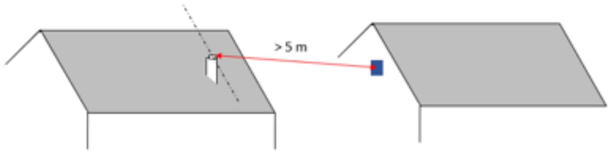
Figure 15 : Distance au bâtiment voisin
