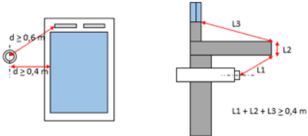
Figure 2 : Position du terminal horizontal des systèmes individuels
